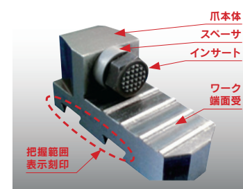
ワークに合わせた数種類のインサート爪をご準備頂ければ、爪の初期成形も不要になります。
