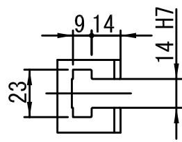
T溝詳細図 X スケール 2 : 5
