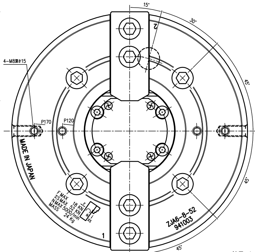
SPECIFICATIONS 油圧チャック仕様
