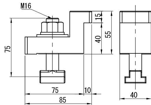
押さえブロック 4ヶ付属
