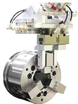
チャックの爪交換
