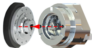
チャック交換
