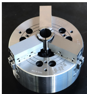
チャックの爪交換+コレット
