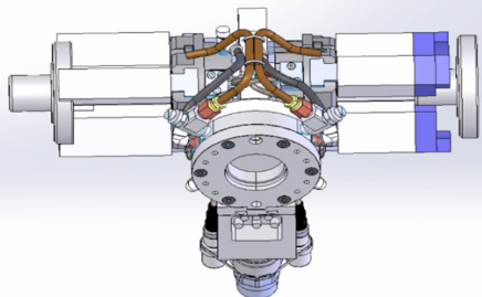
ダブルハンド LG-6 把握力 1000Nm
