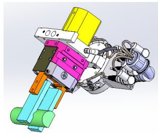
Dカット材把握
