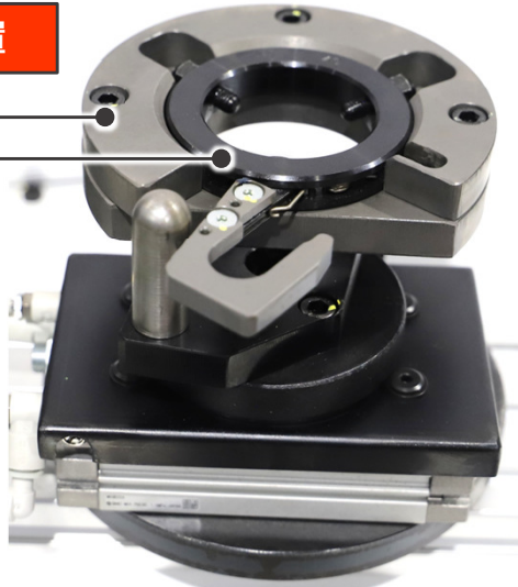
ケレ自動交換装置
